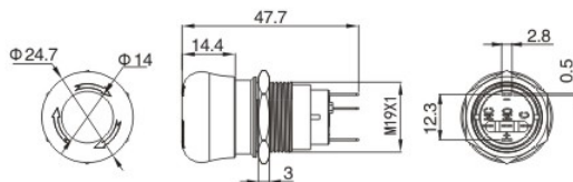
外形尺寸
